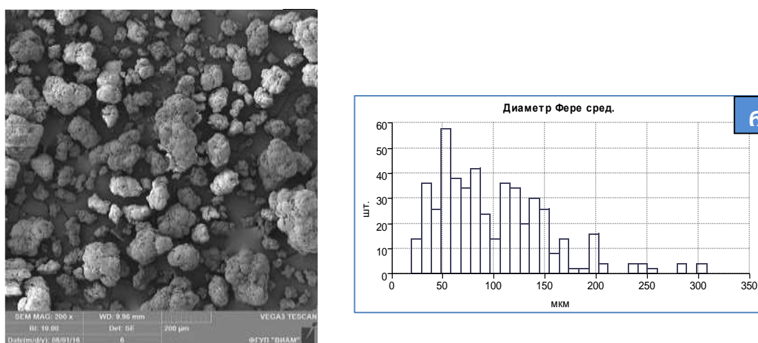
Рис.1 – Микроструктура (а) и гистограмма (б) распределения по размерам частиц порошка Rilsamid AMNO TLD, D_{ср} = 94,7 мкм
