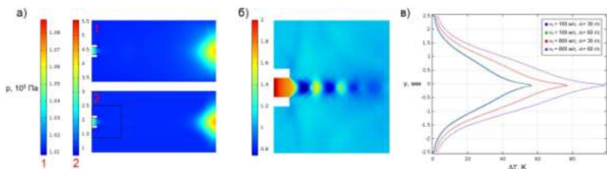
Рис. 5 – а) Распределение давления в газе при скоростях газа 100 м/с (1) и 800 м/с (2), правый край – обрабатываемая поверхность; б) Давление в сверхзвуковой струе при скорости истечения 800 м/с (увеличенная область вблизи сопла); в) Профили температуры обрабатываемой поверхности (указана, как разность конечной и начальной температуры)
