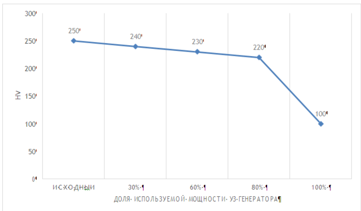
Рис. 4 - Сравнение твердости образцов
