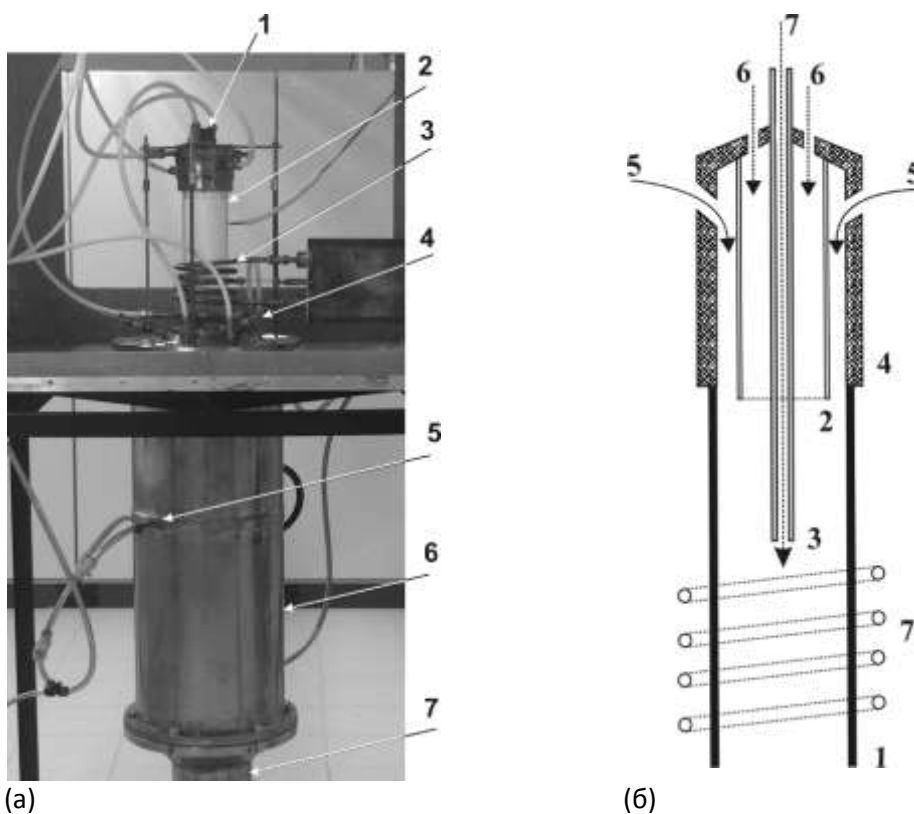
Рис.1. - Конструкция плазмохимического реактора для плазменной обработки порошковых материалов (а): 1 – ввод шихты в начало плазменного факела; 2 – кварцевый плазматрон; 3 – индуктор; 4 – ввод шихты в конец плазменного факела; 5 – подача охлаждающего газа; 6 – конденсационная камера; 7 – выход готового порошка;
