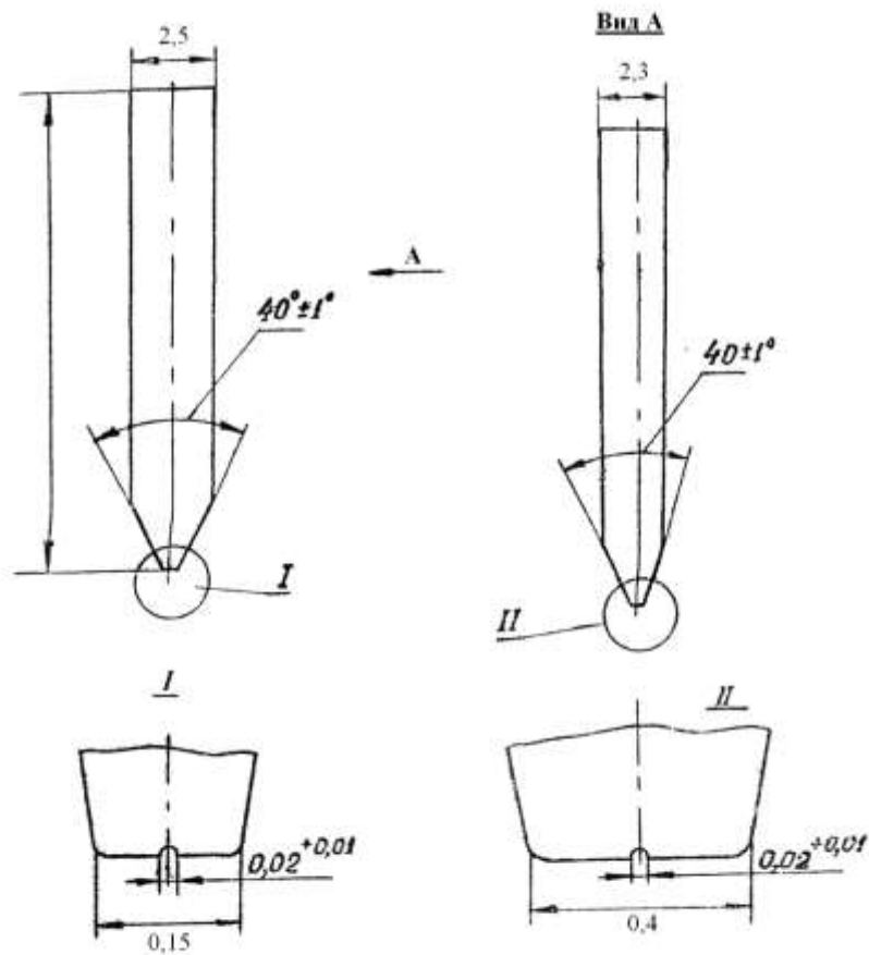
Чертеж 2. Инструмент игольчатый для УЗС с рабочей частью \varnothing 0,3 мм.
