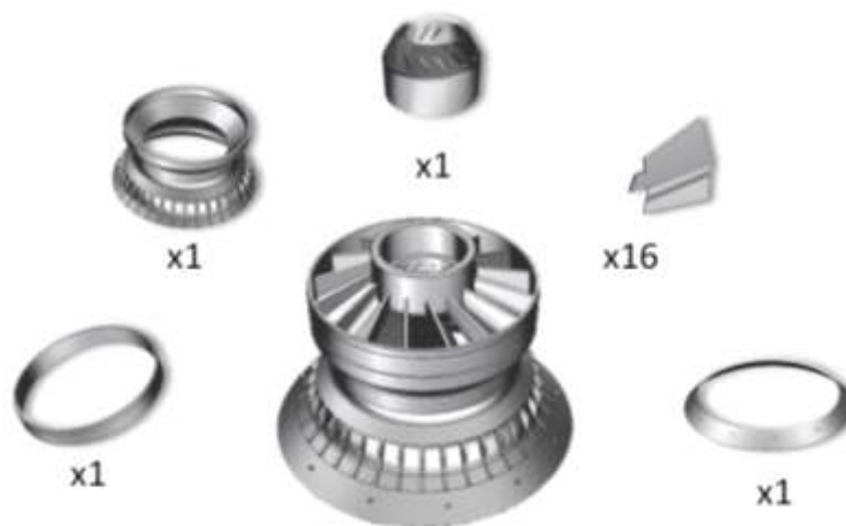
Рис. 5 – Центральный завихритель и входящие в его состав ДСЕ
