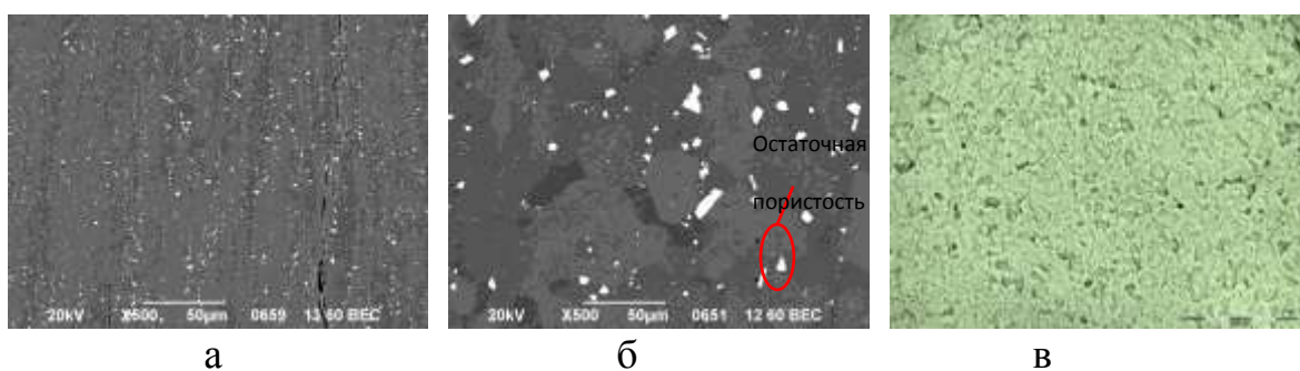
Рисунок 2 – Микроструктура синтезированного материала после ВТО а) ( T_S-30 )°С, РЭМ, б) ( T_S-10 )°С, РЭМ, в) ( T_S-10 )°С, СМ
