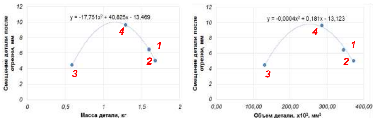
Рисунок 1 – Влияние массы и объёма деталей на её коробление
