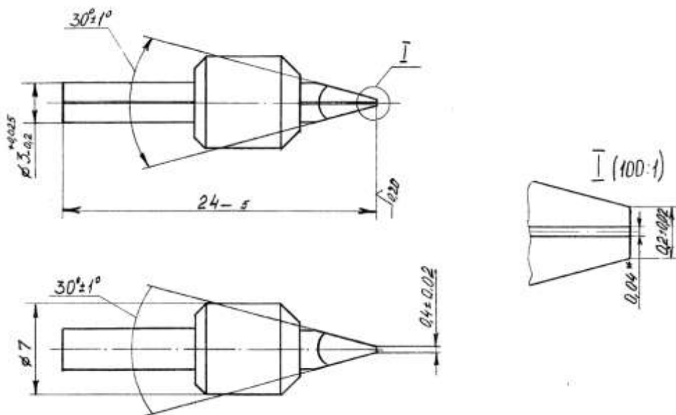
Чертеж 1 - Расщепленный электрод для МКТС
