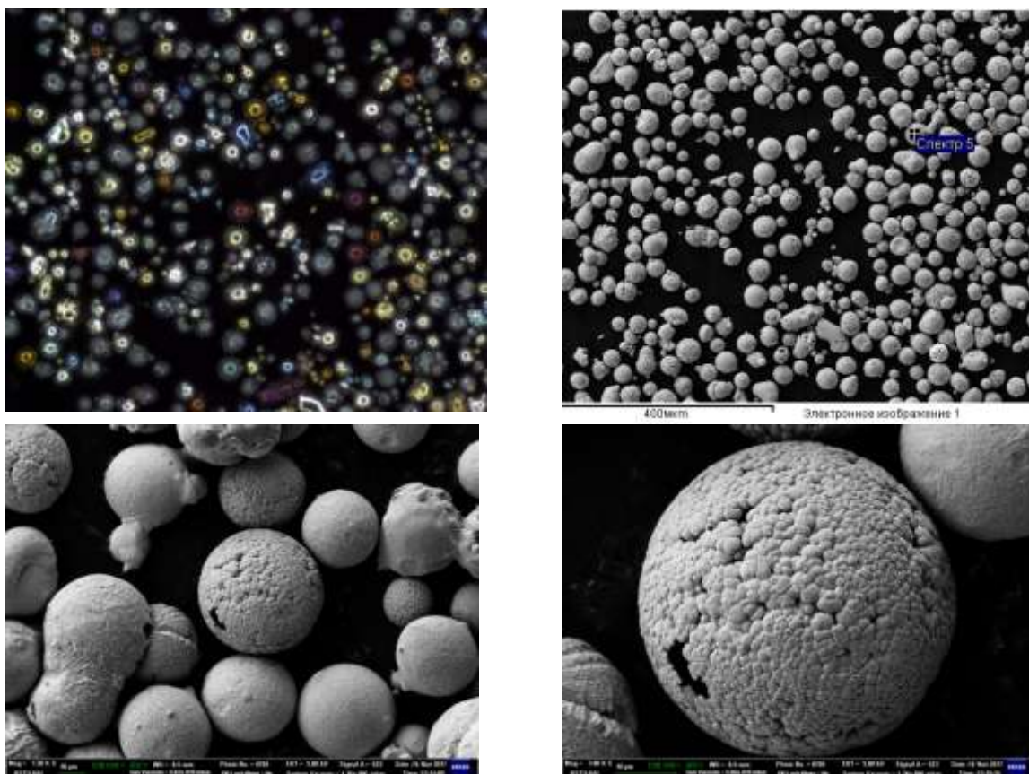
Рис. 4 - SEM-изображения частиц обработанного порошка.
