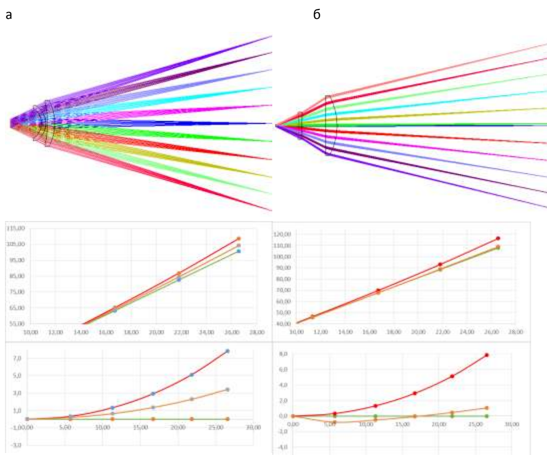
Рис. 4 – Двухлинзовая система
