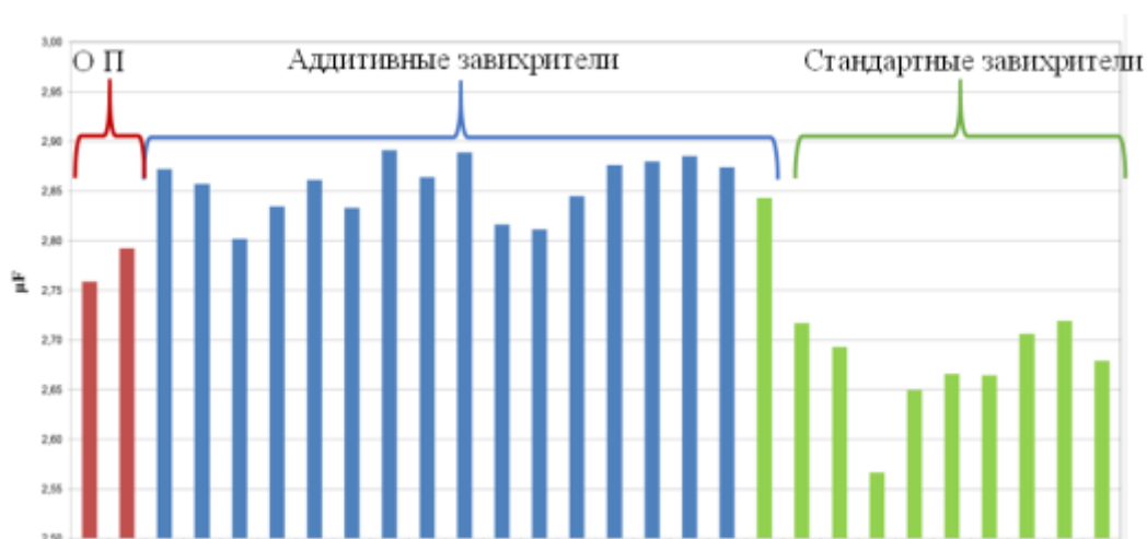
Рис. 3 – Результаты определения расходных характеристик завихрителей
