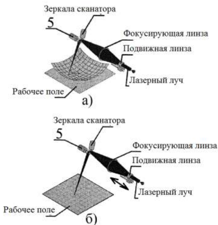
Рис.1 – Плоскость фокуса 2D сканатора (а), 3D сканатора (б)
