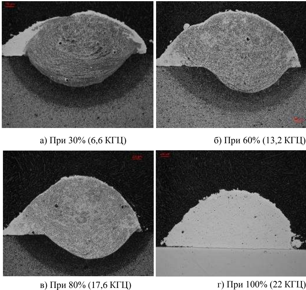
Рис. 3 - Микрофотографии образцов полученных под воздействием УЗ колебаний
