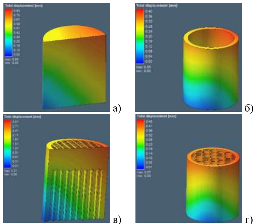
Рисунок 5 - Результаты моделирования в Simufact.Additive
