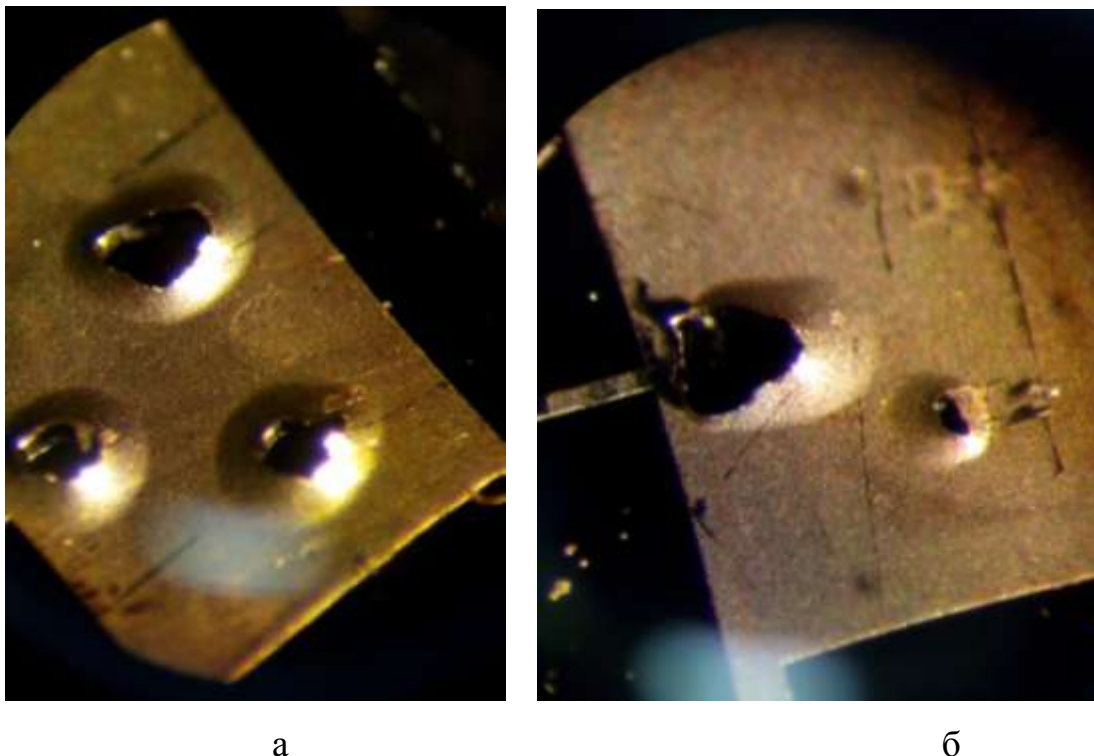
Рис. 6. – Отслоение некачественного серебряного покрытия на ФП из кремния
