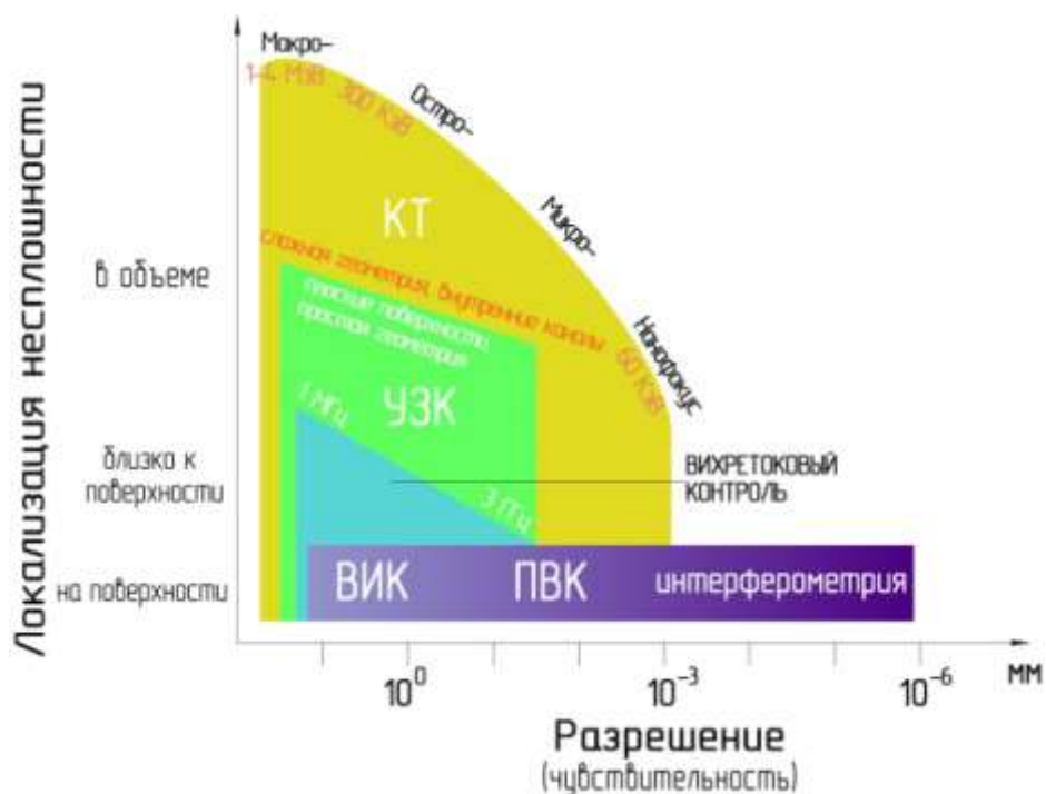
Рис. 1 – Сравнение возможностей методов НК по критерию разрешающей способности в зависимости от местоположения дефекта [7]
