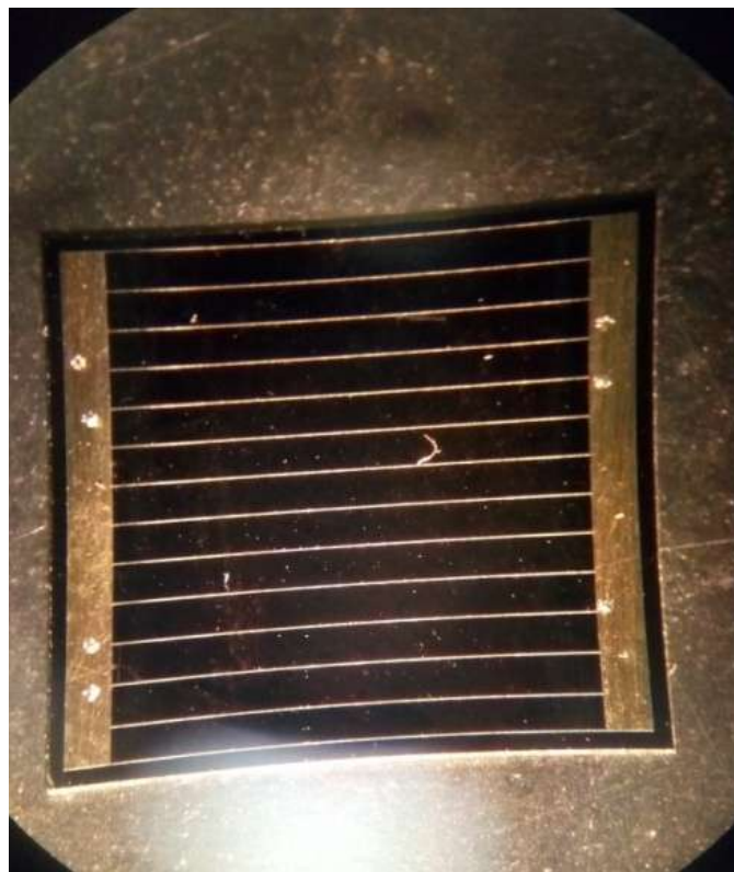
Рис.5. ФП из арсенида галлия 10x10мм
