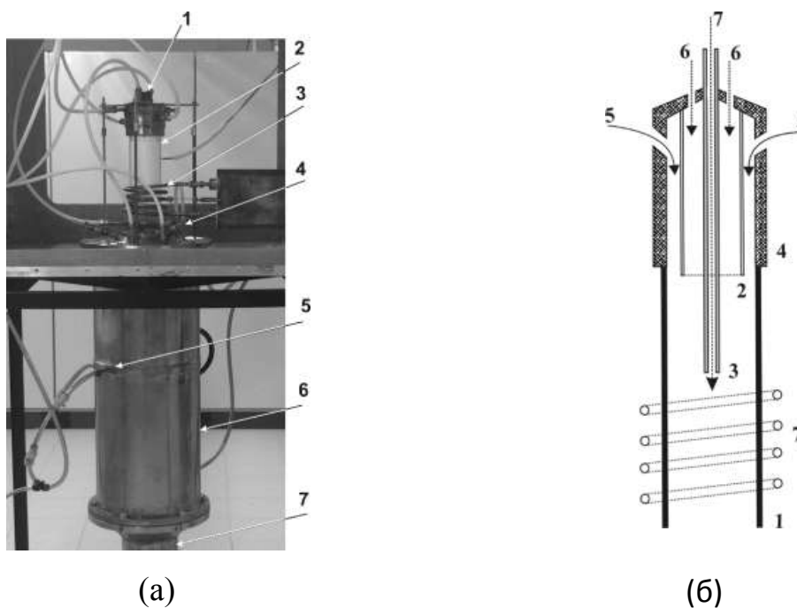
Рис. 1 - Конструкция плазмохимического реактора для плазменной обработки порошковых материалов (а): 1 – ввод шихты в начало плазменного факела; 2 – кварцевый плазматрон; 3 – индуктор; 4 – ввод шихты в конец плазменного факела; 5 – подача охлаждающего газа; 6 – конденсационная камера; 7 – выход готового порошка. Кварцевый плазматрон (б): 1- внешняя кварцевая трубка; 2 – промежуточная кварцевая трубка; 3 – порошковый питатель; 4 – завихритель; 5 – подача защитного газа; 6 – подача плазмообразующего газа; 7 – подача транспортного газа; 8 – индуктор.
