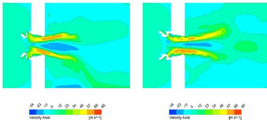
Распределение осевой скорости воздушного потока на режиме \Delta P = 0,03 \text{ кг/см}^2
