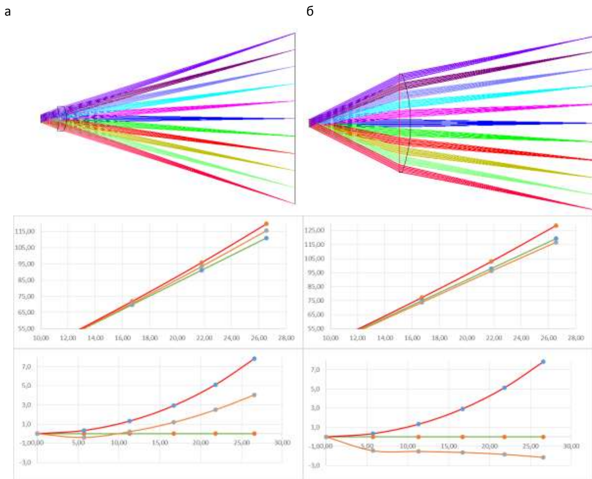
Рис. 3 – Однолинзовая система
