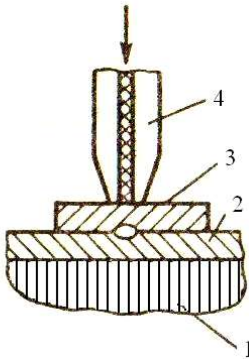
1 – ФП; 2 – Серебряная контактная площадка ФП; 3 – Серебряный токовывод; 4 – Сдвоенный (расщепленный) электрод.
