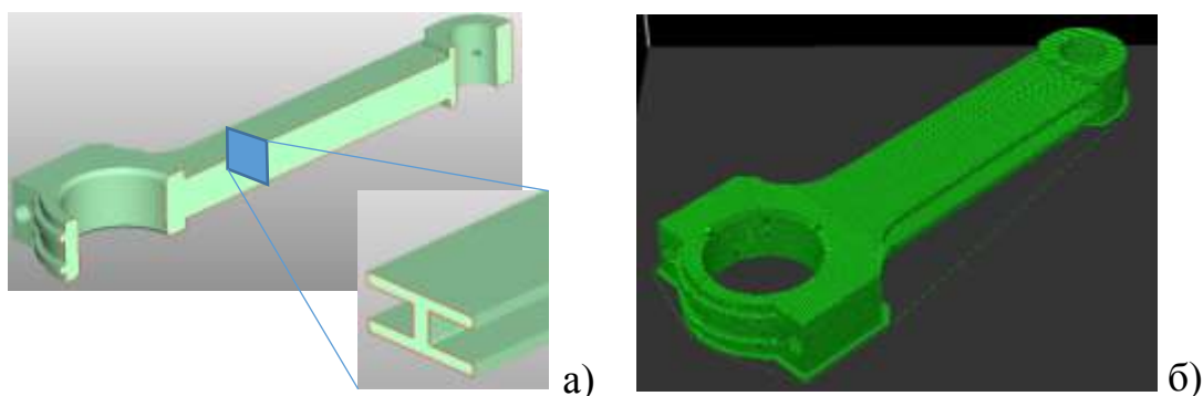
Рисунок 2 – Исходная 3D-модель детали «Шатун» (а) и подготовленные gcode (б)
