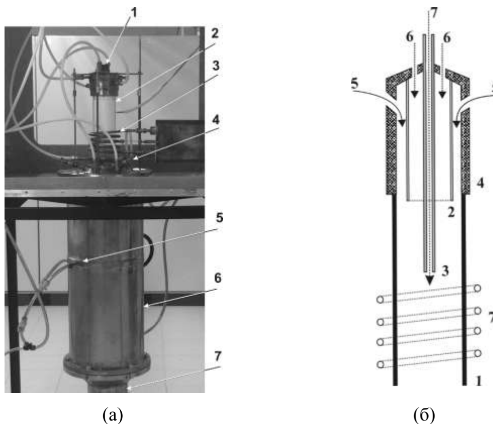
Рис.1. - Конструкция плазмохимического реактора для плазменной обработки порошковых материалов (а): 1 – ввод шихты в начало плазменного факела; 2 – кварцевый плазматрон; 3 – индуктор; 4 – ввод шихты в конец плазменного факела; 5 – подача охлаждающего газа; 6 – конденсационная камера; 7 – выход готового порошка. Кварцевый плазматрон (б): 1- внешняя кварцевая трубка; 2 – промежуточная кварцевая трубка; 3 – порошок питатель; 4 – завихритель; 5 – подача защитного газа; 6 – подача плазмообразующего газа; 7 – подача транспортного газа; 8 – индуктор.
