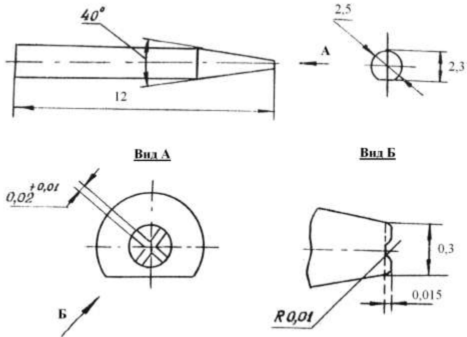
Чертеж 2. Инструмент игольчатый для УЗС с рабочей частью \varnothing 0,3 мм.
