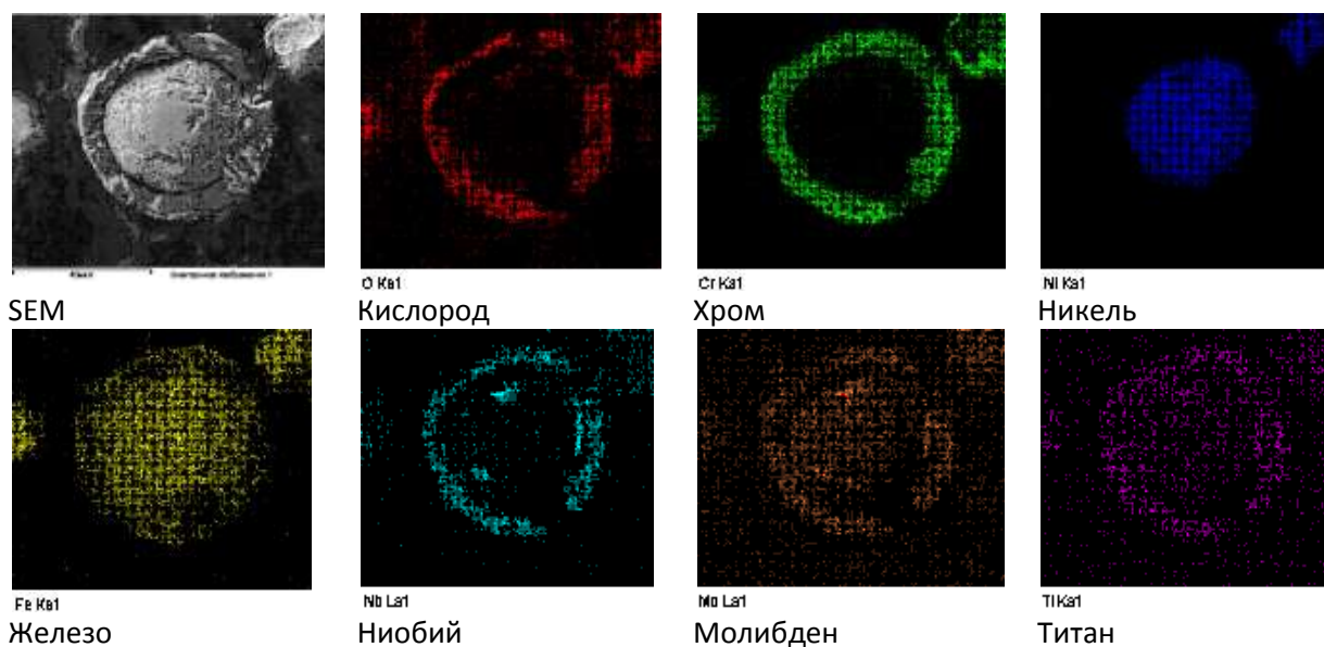
Рис. 5 - Энерго-дисперсионный анализ частицы обработанного порошка
