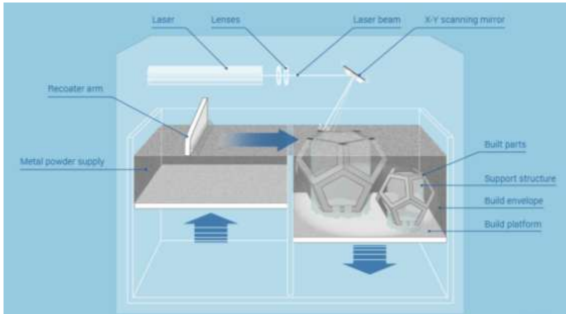
Рис. 1 – Процесс аддитивного производства методом селективного лазерного плавления
