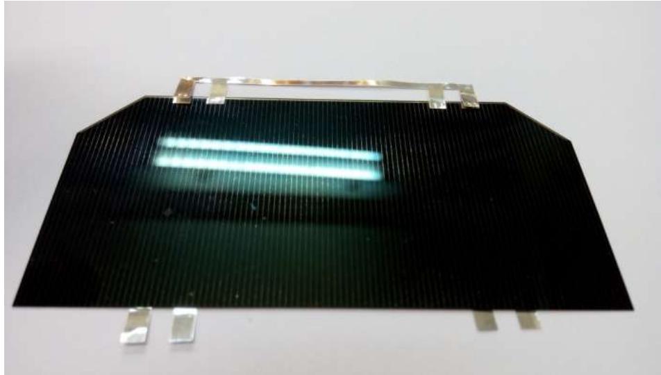
Рис.4. ФП из арсенида галлия 37x76 мм
