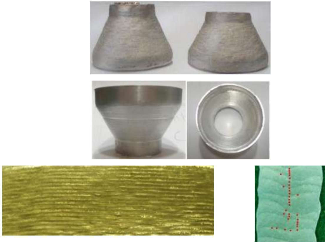
Рис. 7 – Патрубки из сплава АМг5 полученные по аддитивной технологии дуговой наплавкой до и после мехобработки. Диаметр 35–60 мм, толщина стенки 5 мм.
