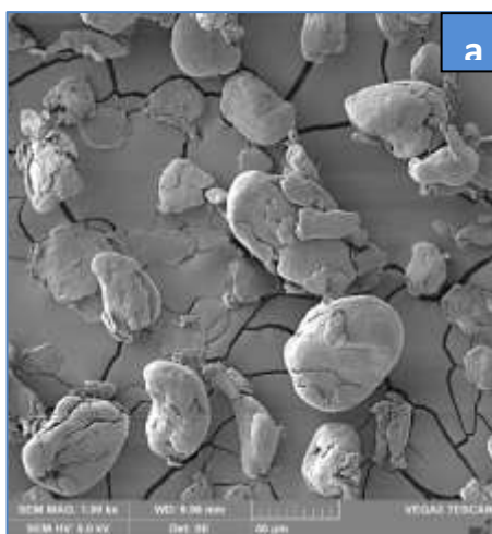
Рис. 12 – Микроструктура (а) и гистограмма (б) распределения по размерам частиц порошка полиэфирэфиркетона марки Zureek 550 UPF (производитель Китай): D_{cp} = 40,3 \text{ мкм}
