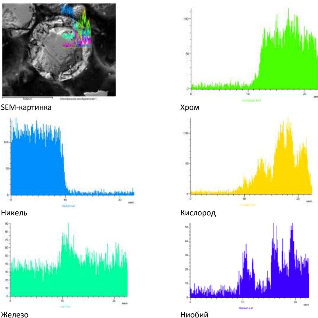
Рис. 6 - Радиальное распределение элементов в сечении частицы порошка
