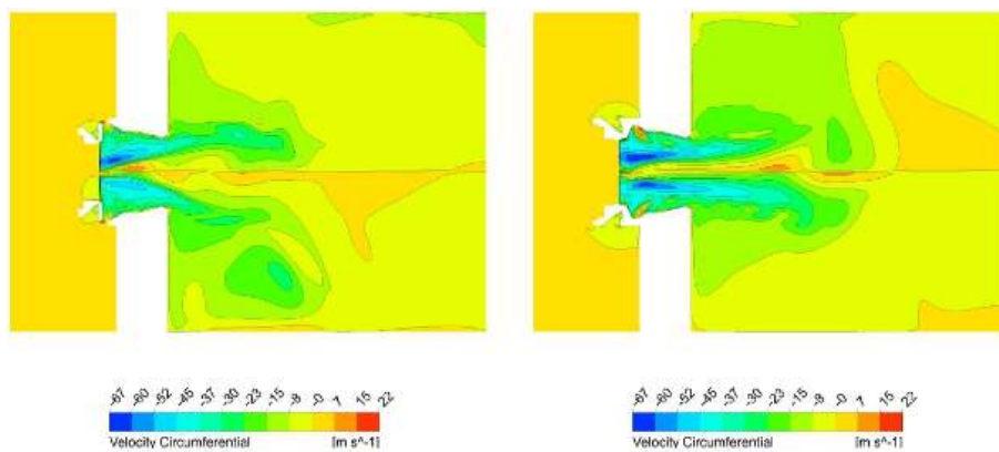
Распределение окружной скорости воздушного потока на режиме \Delta P = 0,03 \text{ кг/см}^2
