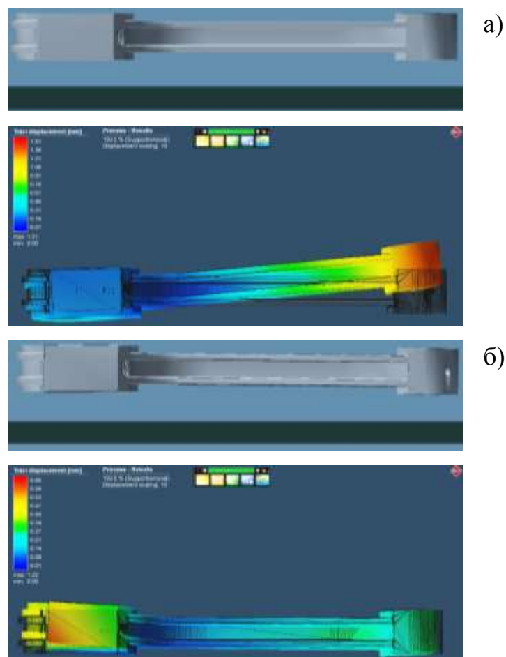
Рисунок 3 - Результаты моделирования в Simufact. Additive
