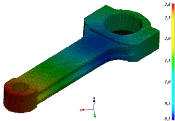
Рисунок 4 - Результаты моделирования в Digimat-AM
