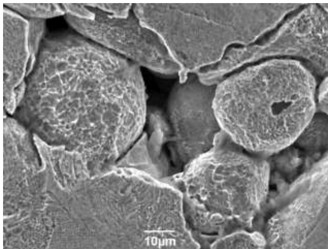
Рис. 5 - Сфероидизация стали 316L при лазерном плавлении
