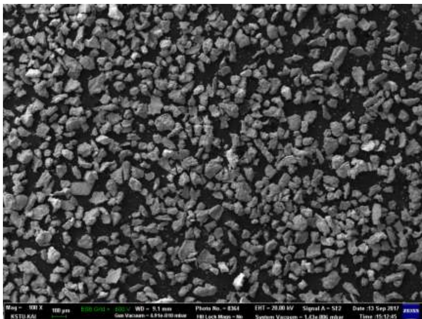
Рис. 2 - SEM-изображение исходного порошка ZrO_2 , стабилизированного Y_2O_3 .
