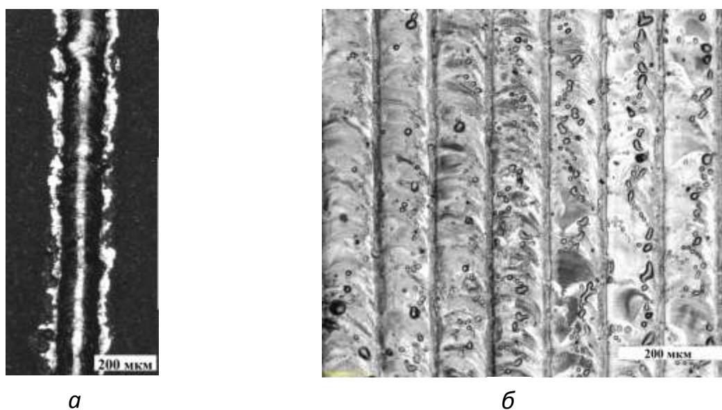
Рис. 1 - Образцы: (а) одиночный валик; (б) единичный слой
