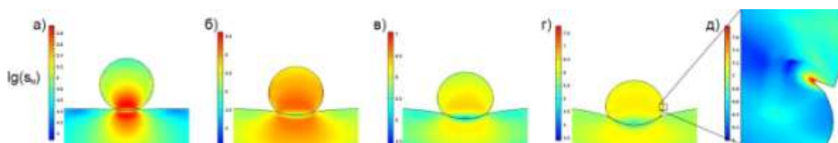
Рис. 4 – Логарифм напряжений по Мизесу в частице и подложке, выраженных в Па для различных скоростей частицы на выходе из сопла Лаваля: а) 100 м/с; б) 600 м/с; в) 700 м/с; г) 800 м/с. д) Увеличенная область посередине частицы
