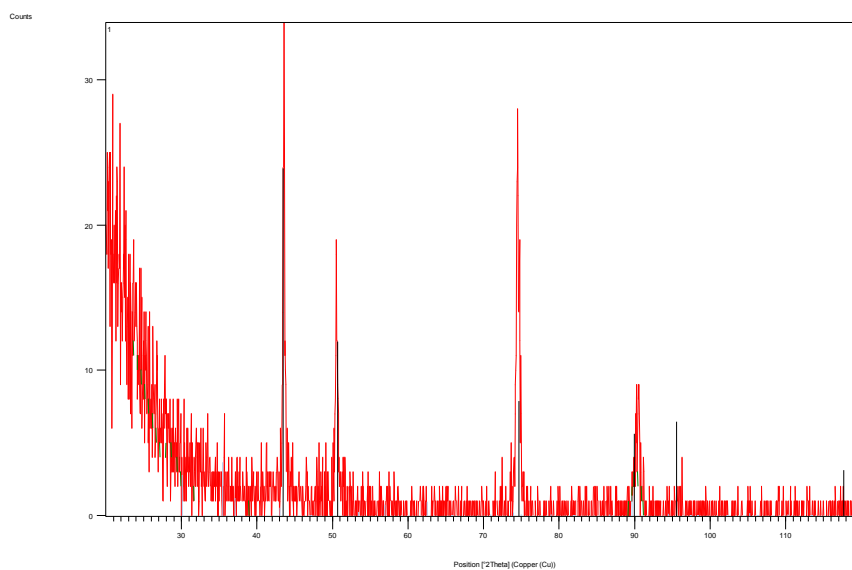
Рис 4 - Дифрактограмма стали 316L, полученной методом селективного лазерного плавления
