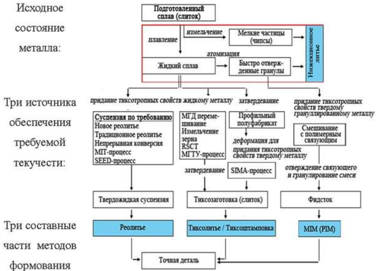
Рис. 2 – Процессы металлургии современных тиксотропных материалов
