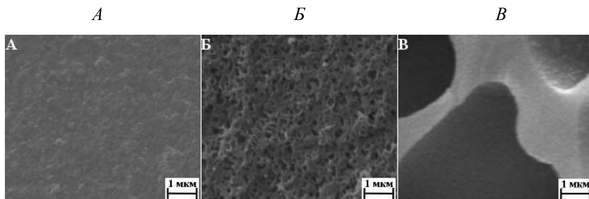
Рис.3 – Микроструктура пиролизатов, полученных на основе различных композиций после проведения стадии МРИП при температуре 60°C: А – мКФЭТ; Б - ФФЭТ; В – пКФЭТ
