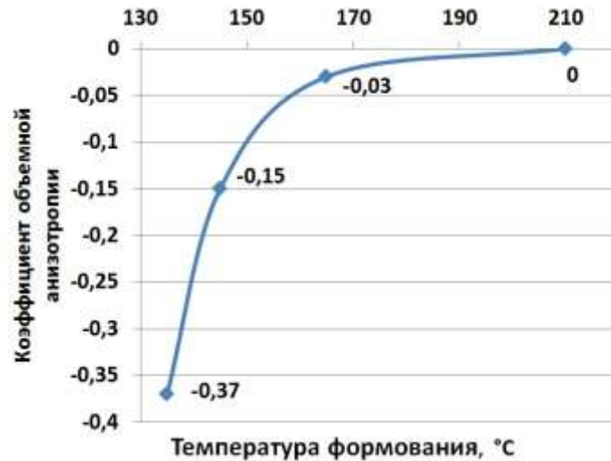
Рис. 6 – Изменение коэффициента объемной анизотропии в образцах из связующего РС-Н
