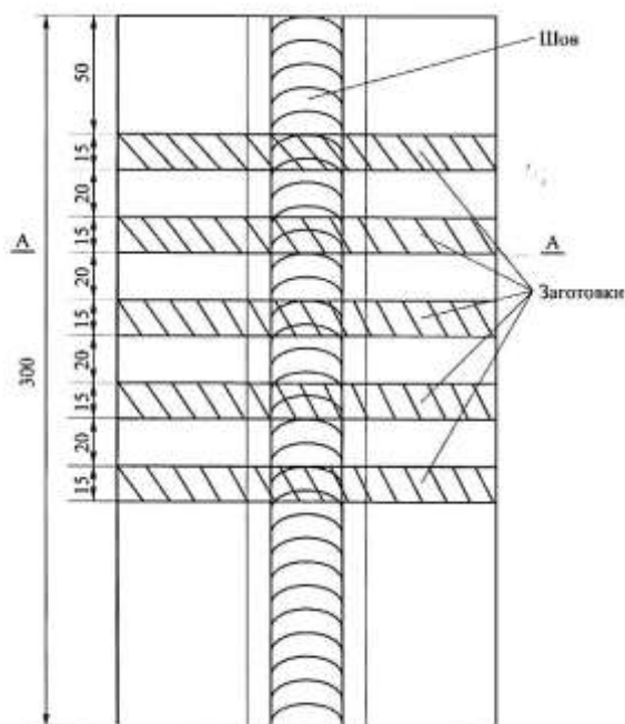
Рис. 2 – Схема вырезки проб для контроля горячих трещин
