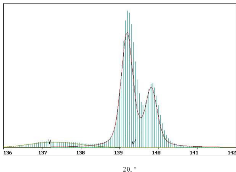
Рис. 1 – Типичная рентгенограмма \gamma/\gamma' -фаз интерметаллидного сплава на основе \text{NiAl} : рефлекс (222) в \text{FeK}_\alpha – излучении
