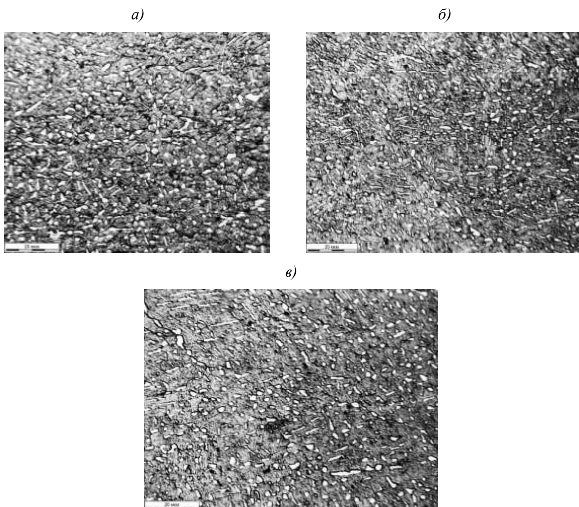
Рис. 2 – Микроструктура сплава VT23. Закалка с 850°C в воде, старение 10 ч. при 550°C-СТО (а), СТО+АТАО1 (б), СТО+АТАО2 (в)
