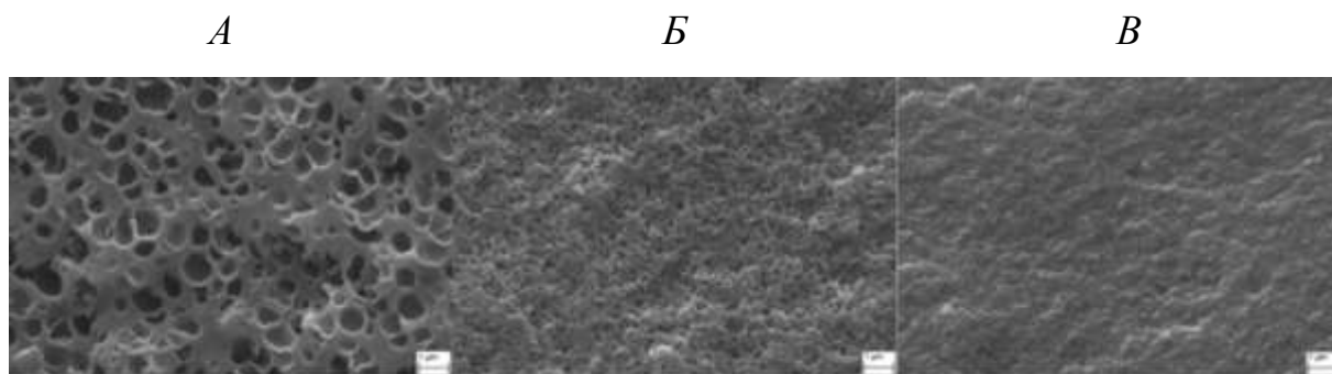
Рис.1 – Микроstructure отвержденных образцов, полученных на основе композиции ФФЭТ после проведения стадии МРИП при различных температурах: А – 50^\circ\text{C} ; Б – 60^\circ\text{C} ; В – 70^\circ\text{C} [1]
