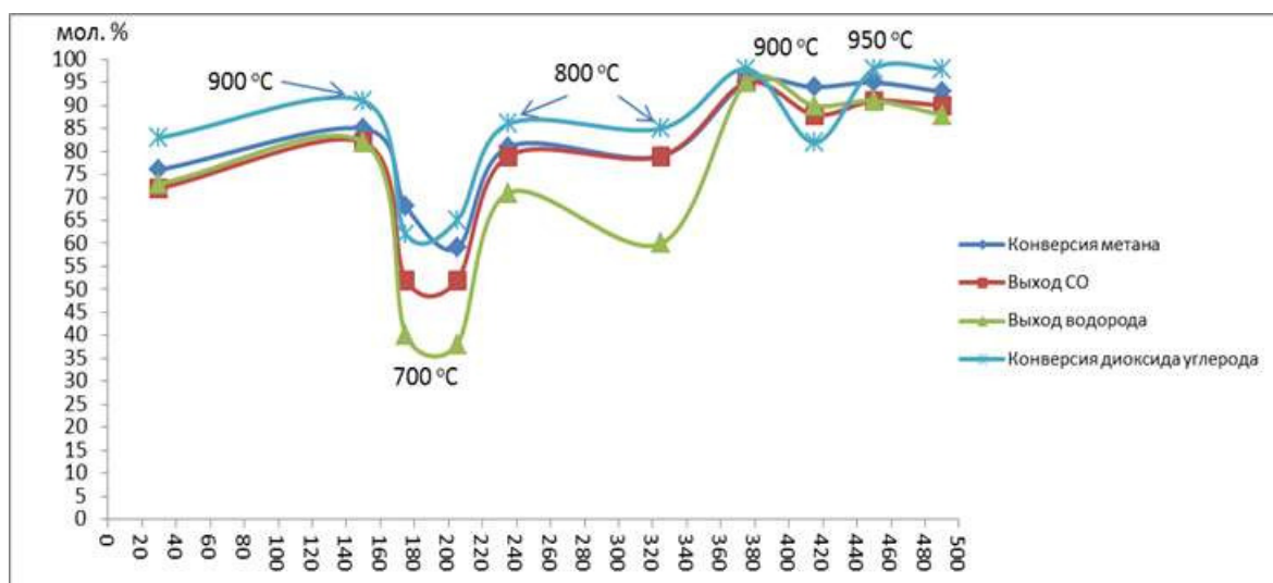
Рис. 6 – Температурная зависимость эффективности катализатора \text{Ru}(\text{CwGm})_3(\text{Вн-С}_4\text{Н}_9)_2@ТЗМК
