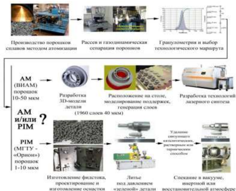
Рис. 5 – Два маршрута изготовления детали «Завихритель»
