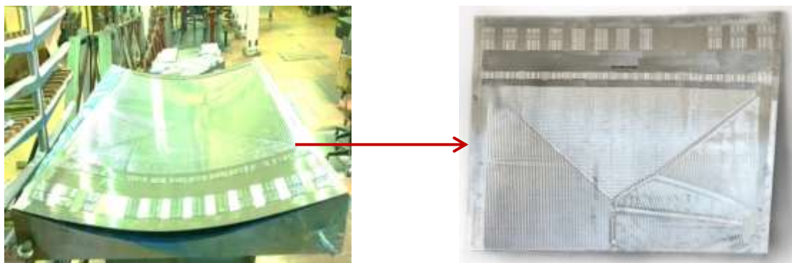
Рис. 8 – Формообразованная деталь из листа сплава В95очТ2, установленная на технологическую матрицу
