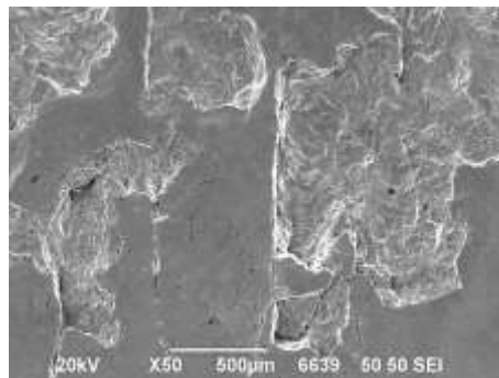
Рис. 4 – Наружное кольцо подшипника № 2. а – следы абразивного изнашивания на внешнем диаметре наружного кольца; б – выкрашивания на дорожке качения; в, г – трещины и выкрашивания на дорожке качения
